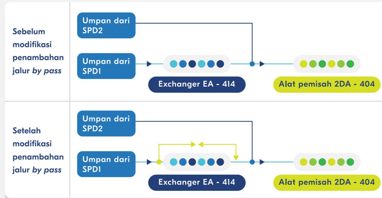
Gambar 6. Skema modifikasi penambahan jalur By pass
